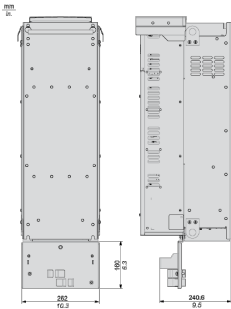
Desenhos da esquerda para a direita: vista traseira, vista lateral direita com tampa superior.
