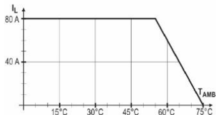
Figura 4 – SSR4880 + dissipador NDP3-120 mm + Ventilador 3 m/s
