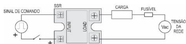
Figura 2 – Conexões Elétricas – Sinal de comando e carga
