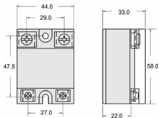
Figura 7 – Dimensões do SSR
