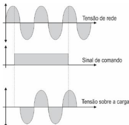
Figura 1 – Tensão elétrica sobre uma carga resistiva
