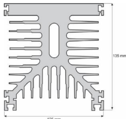
Figura 6 – Dissipador NDP3 (para 120 mm: R thja = 0,52 °C / W)
