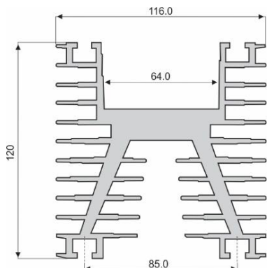
Figura 5 – Dissipador ND40 (para 100 mm: R thja = 0,65 °C / W)
