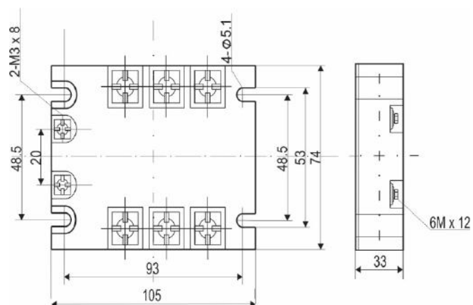
Fig. 5 – Dimensões do SSR
