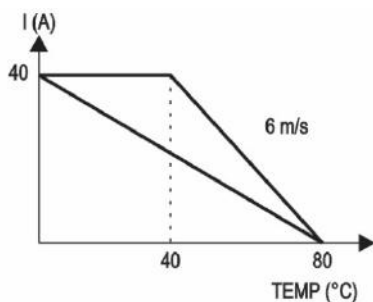
Fig. 3 - SSR3-4840 com dissipador NDP3-120 mm
