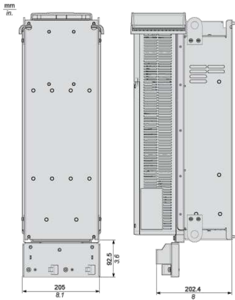
Desenhos da esquerda para a direita: vista traseira, vista lateral direita com tampa superior.
